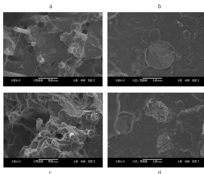
4. ábra. PLA+BF+2MMT próbatétel töretfelülete (x500 (a) és x1000 (b) nagyításban), PLA+BF+2MMT próbatétel töretfelülete (x500 (c) és x2500 (d) nagyításban)
