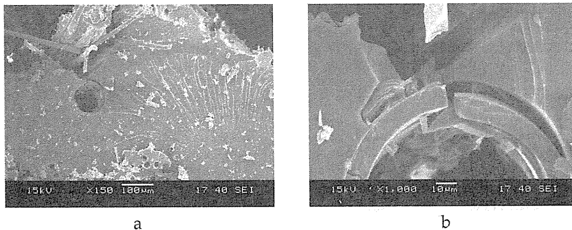
3. ábra. A töret felület (a) és repedt üreges üvegszál nagyított (b) pásztázó elektronmikroszkópos felvétele
