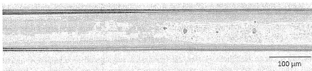
2. ábra. Az üreges üvegszál (kék) feltöltése hidrogén peroxiddal (piros)
